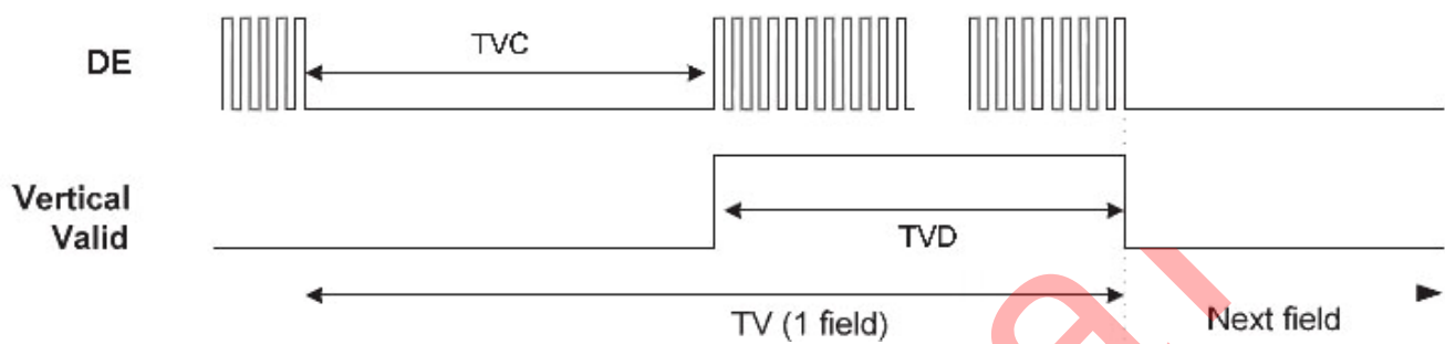
DE Mode Input Timing
